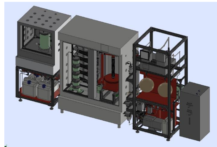
低温CO2回収装置
