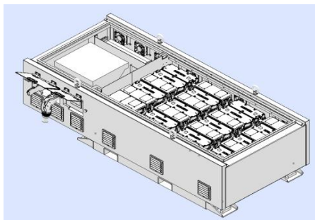
搭載部
