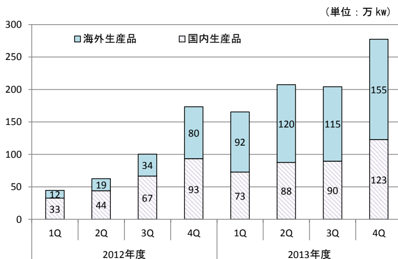
【図表③】日本の太陽電池モジュール出荷量
