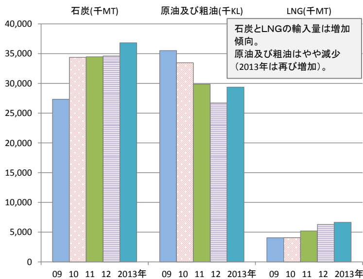
【図表④】九州の主な鉱物性燃料の輸入数量の推移
